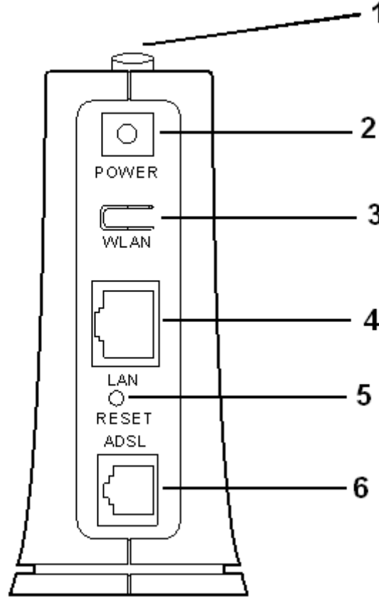
Şekil 1-2. HG521v1 üzerindeki arayüzler ve tuşlar
